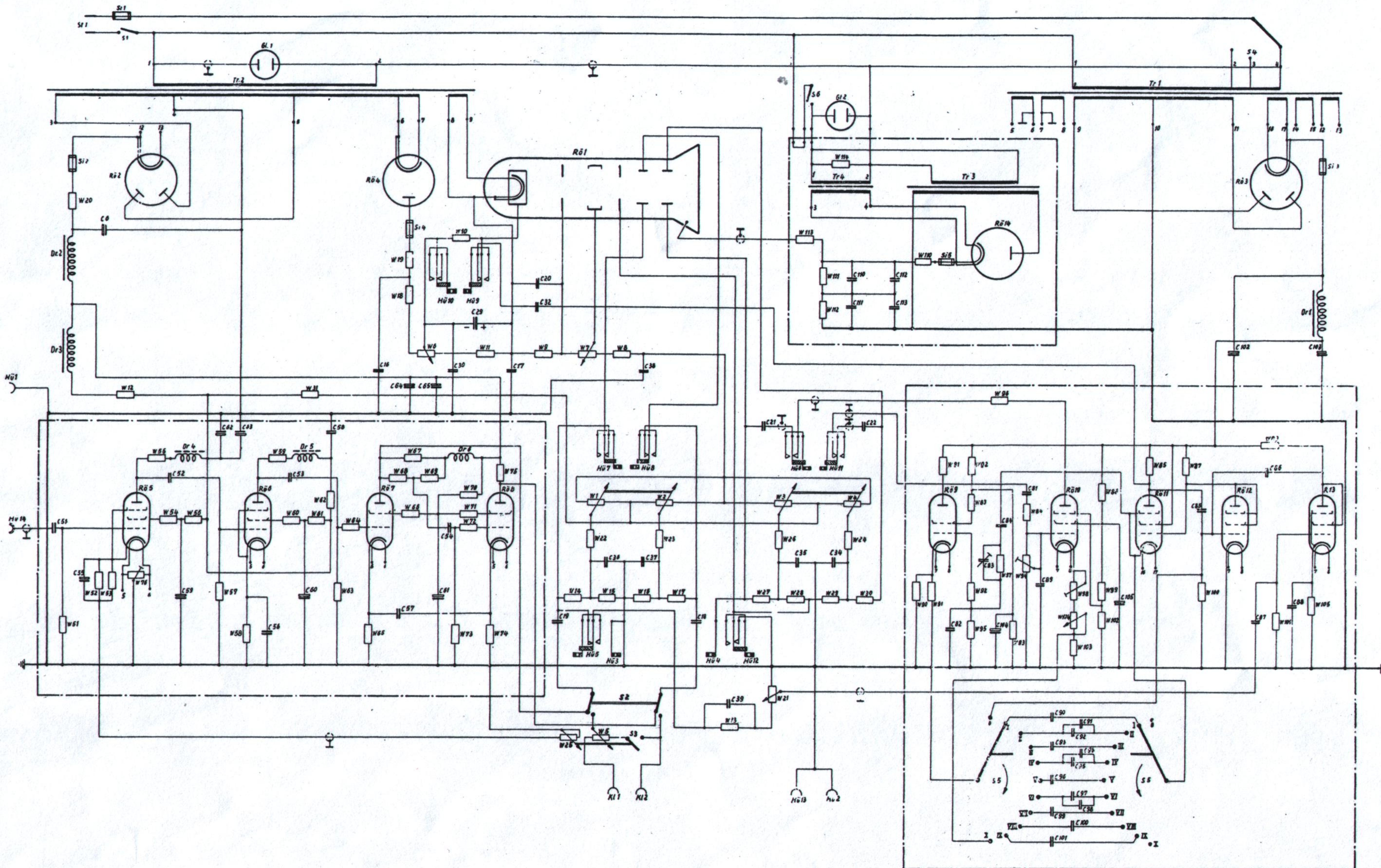
Schaltbild zum Einstrahl-Oszillograf 1 KO - 712
