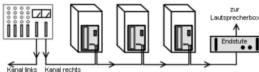
Abb.: A100 in Kette mit nachgeschalteter Endstufe
